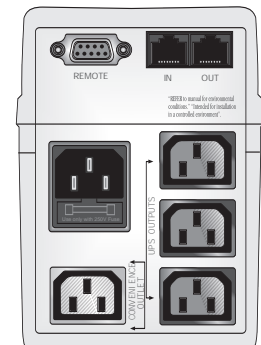
Configuración del Panel trasero
